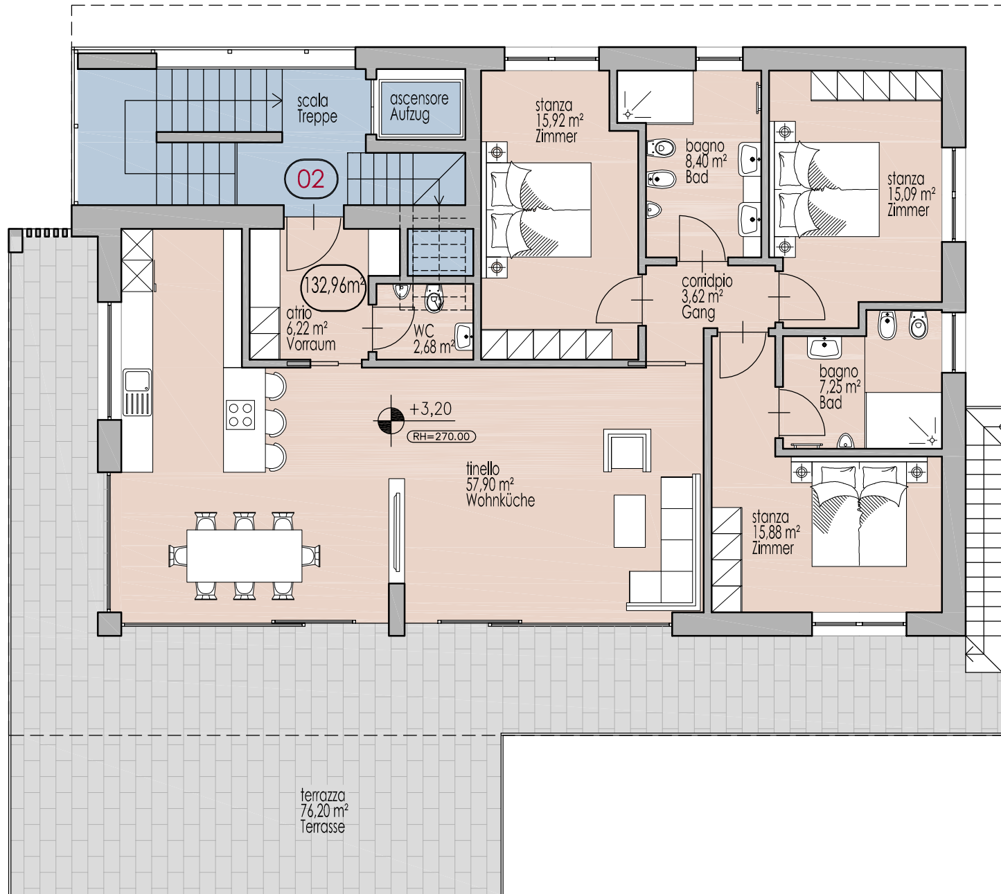
Sottotetto - Dachgeschoss
