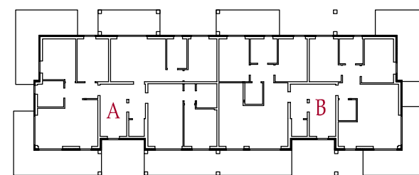
Lageplan - planimetria
