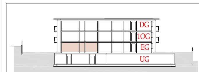
Schnitt - sezione
